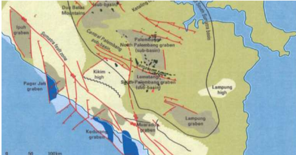
Gambar 3. Wilayah Kota Bengkulu menjadi bagian dari sebaran graben Pagarjati, (Yulihanto, et-al, 1995)
