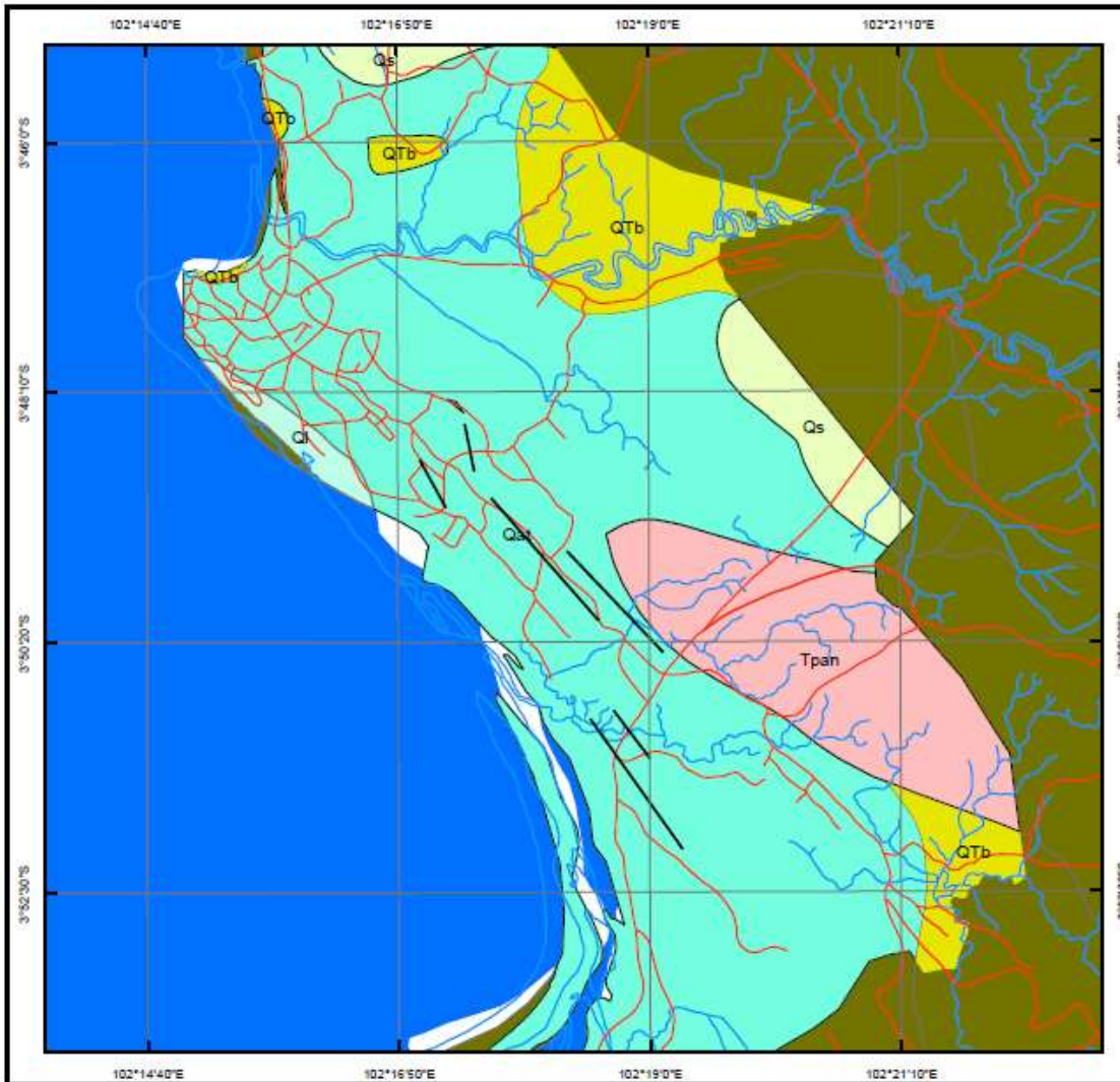
Gambar 4. Peta Geologi Wilayah Kota Bengkulu.
