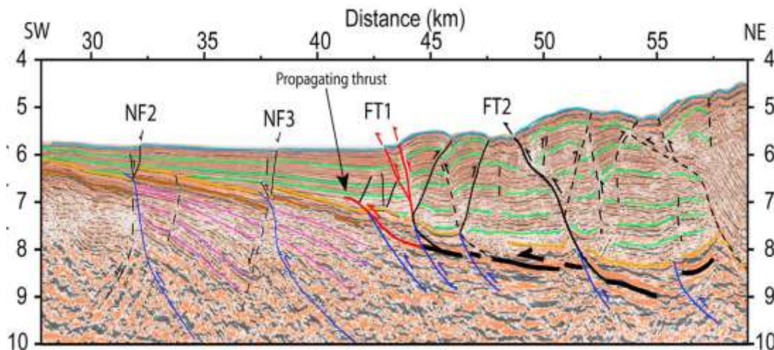
Gambar 2. Penampang seismic refleksi segmen Mentawai pada zona subduksi Sumatra (Singh, et-al, 2010).
