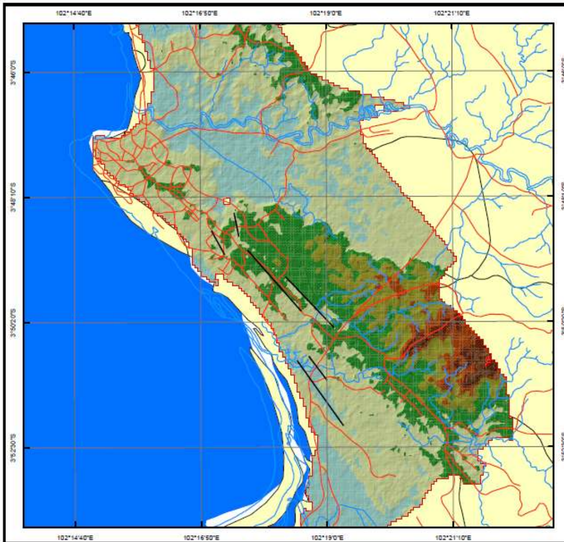
Gambar 5. Peta Struktur Geologi di Wilayah Kota Bengkulu.
