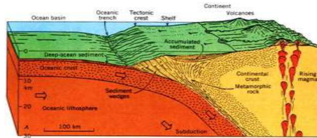
Gambar 1. Penampang zona subduksi Sumatra menurut Kerry Sieh (2003).
